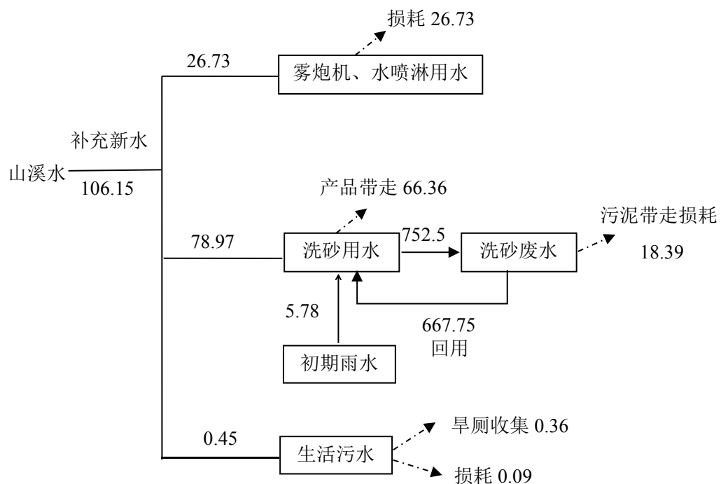
图 2-2 项目水平衡分析图 (m 3 /d)
