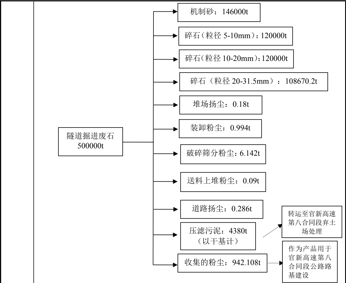
图 2-1 项目物料平衡图
